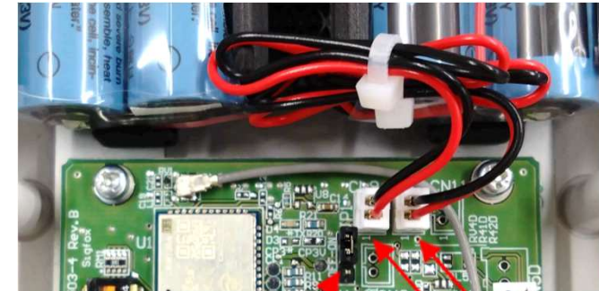
電池コネクタ
